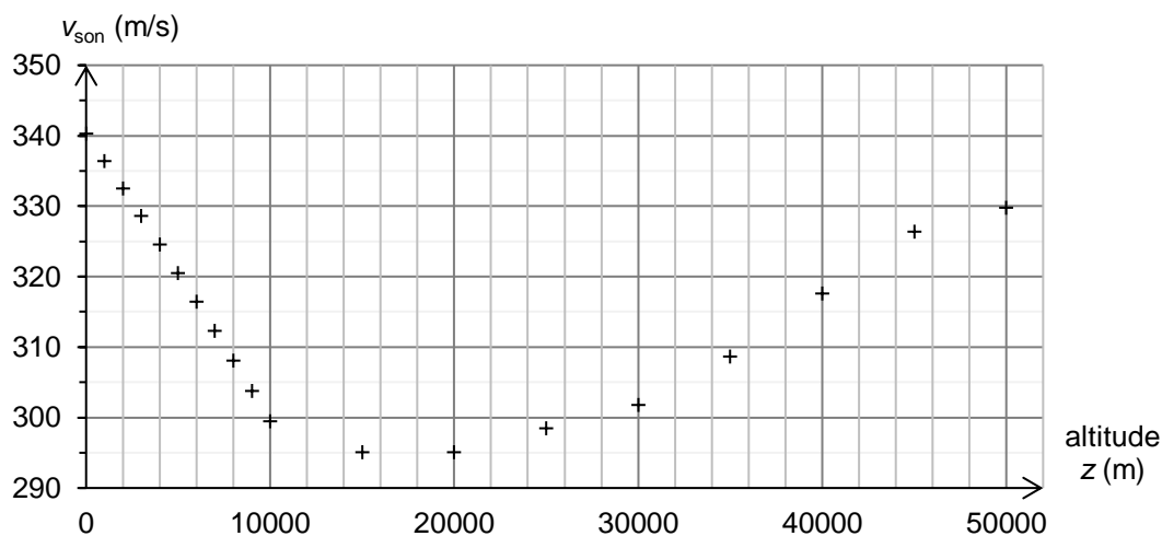
Figure 1. Vitesse du son en fonction de l'altitude
